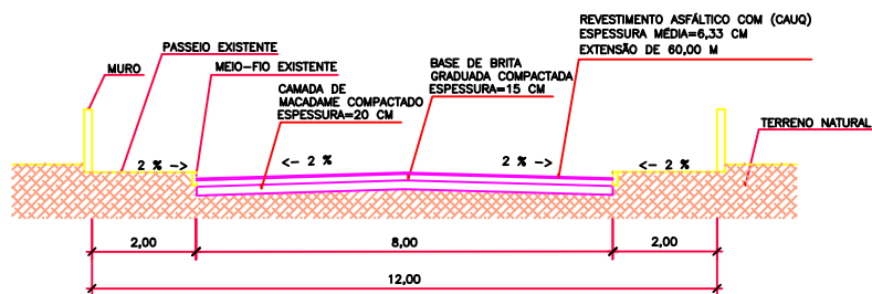
PERFIL TRANSVERSAL
