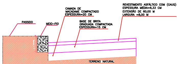
DETALHE DA PAVIMENTAÇÃO
