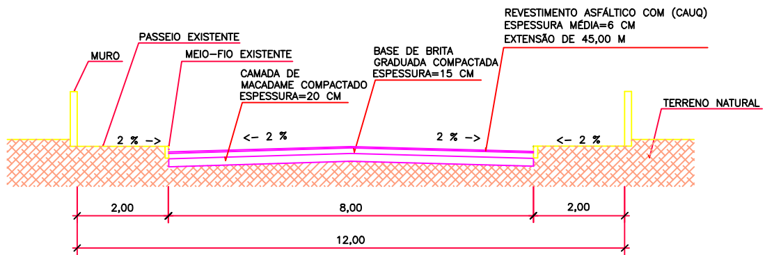
PERFIL TRANSVERSAL
