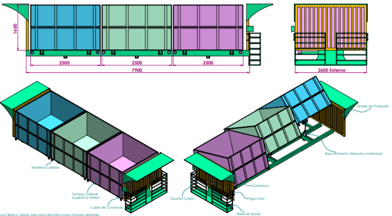
Layout Básico. Seguir Memorial descritivo para maiores detalhes.
